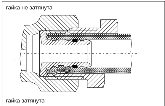
„Sofit S“ присоединительный набор со стяжным кольцом для металлопластиковой трубы, внутренняя резьба
