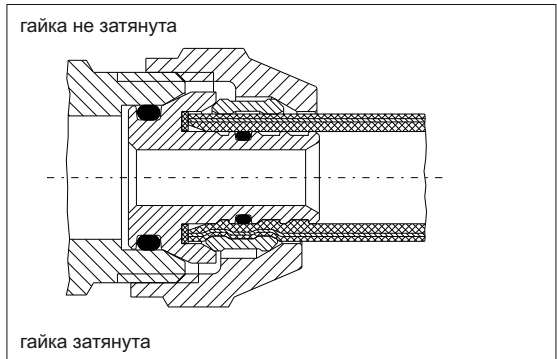
„Sofit S“ присоединительные наборы со стяжным кольцом - универсальное применение для металлопластиковой трубы „Soripe“ и при аналогичной обработке также для полиэтиленовой трубы (PE-X), наружная резьба
