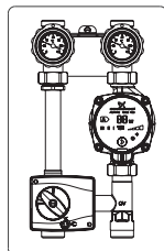
Regumat 130/180 Ду 20/25 арматурные группы с энергоэффективным насосом с или без трехходового смесителя
